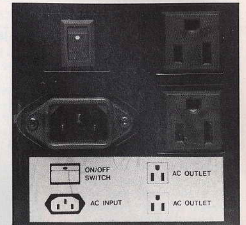
Interrupteur de marche/arrêt, prise secteur, sorties alimentées.
