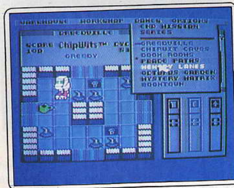
Chipwits
